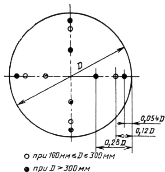
Рисунок 1 - Координаты точек измерения давлений и скоростей в воздуховодах цилиндрического сечения
